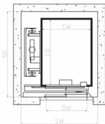
OLT - Oleodynamic 1:2
